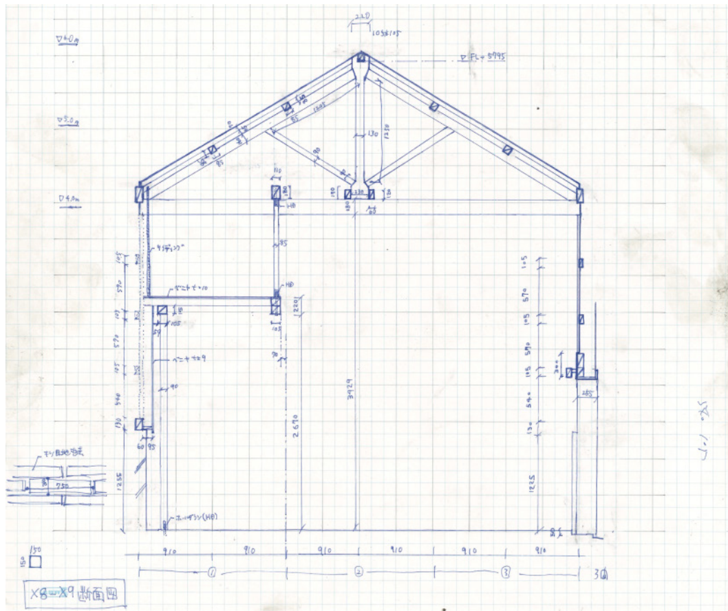
蔵 断面
