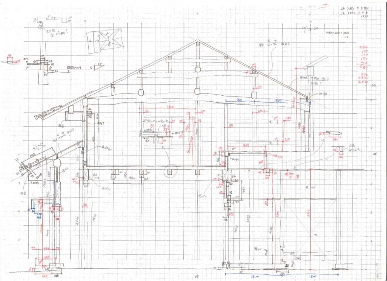
母屋 断面
